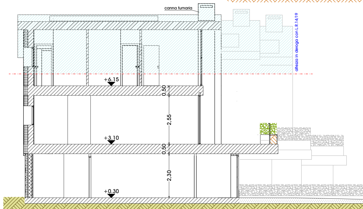
Sezione A-A
