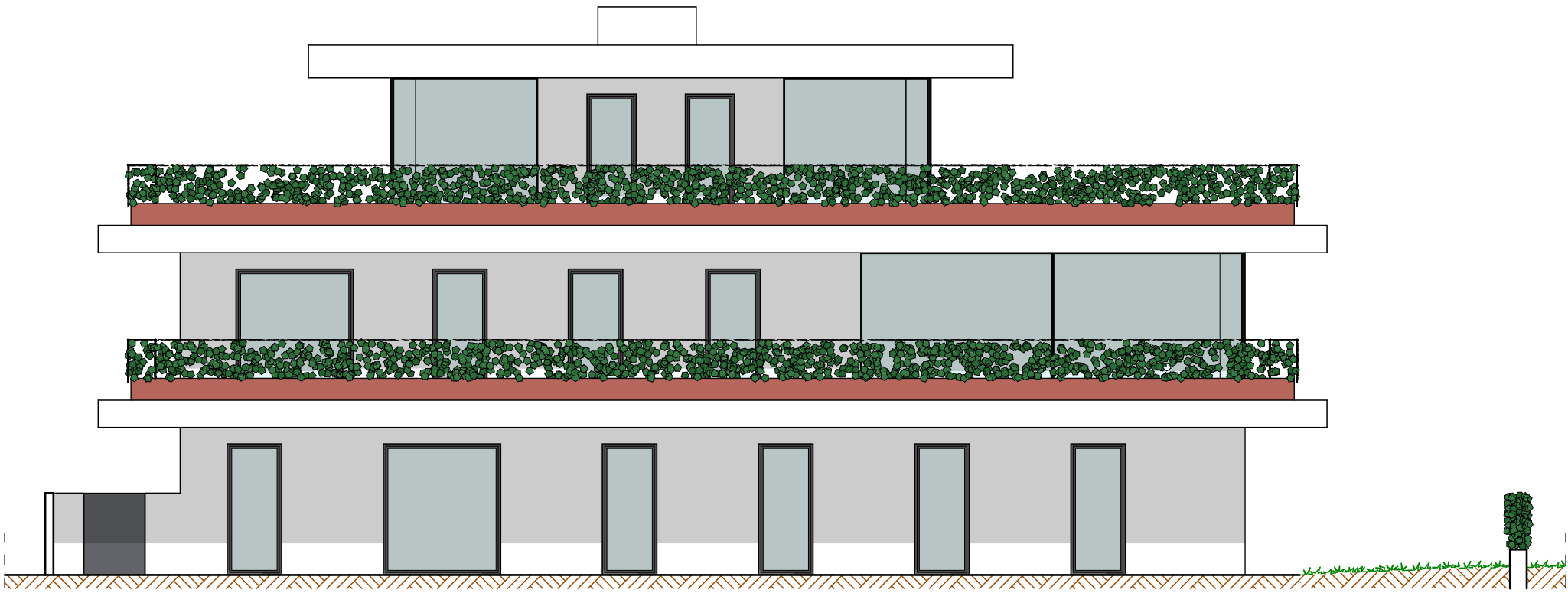
PROSPETTO SUD-EST
